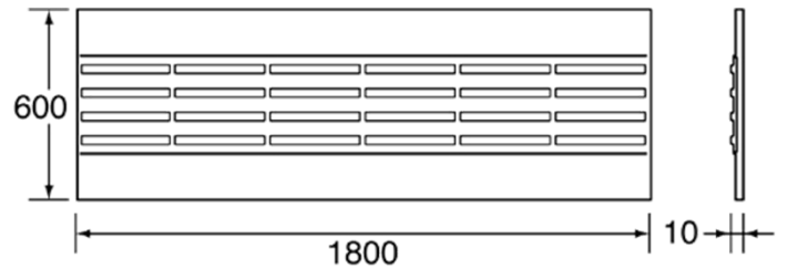
【寸法図】
